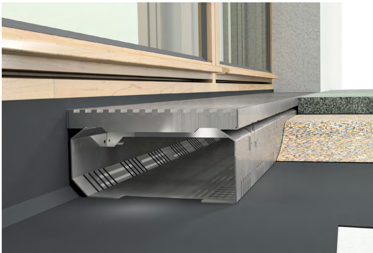
DRAINTEC seitliche Ansicht
