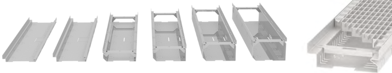
DRAINTEC Rinne in den Bauhöhen 40, 50, 75, 100, 125 und 140 mm
